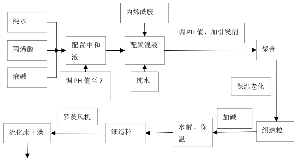
图 4.1-1 聚丙烯酰胺工艺流程框图
