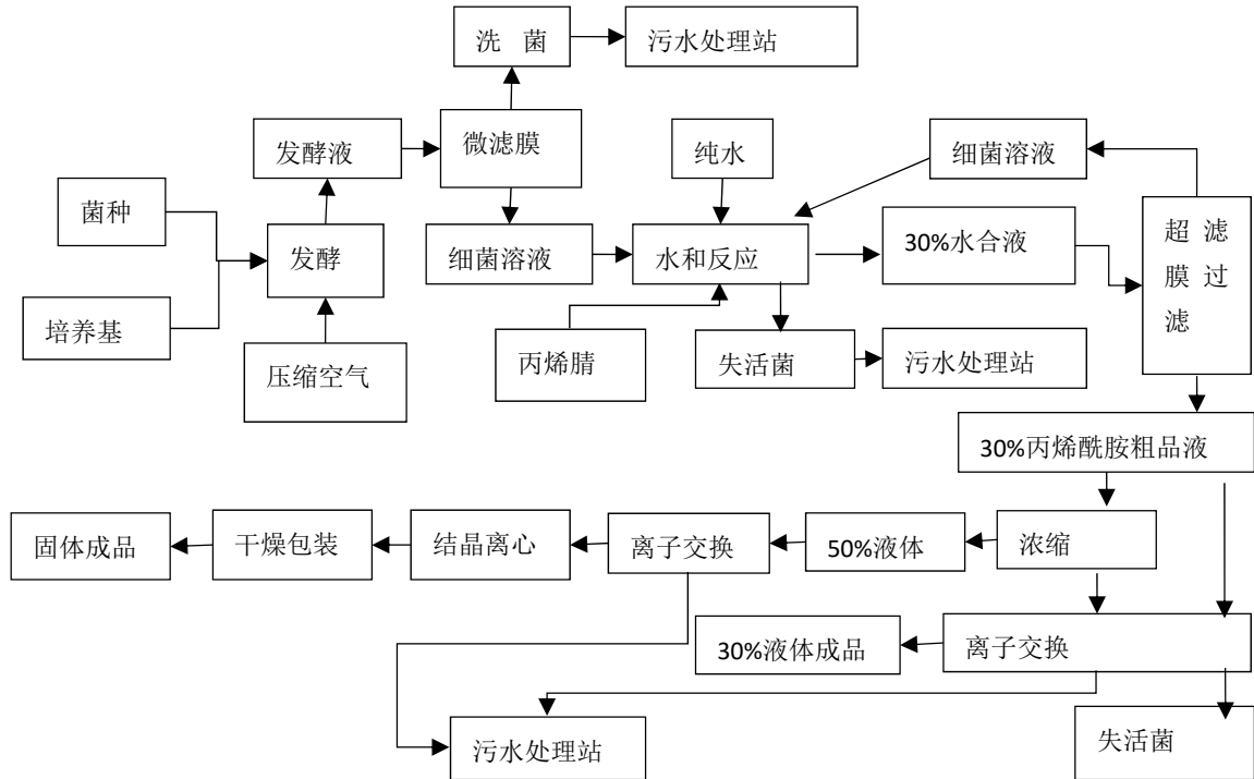
图 4.1-5 丙烯酰胺、丙烯酰胺晶体工艺流程框图
