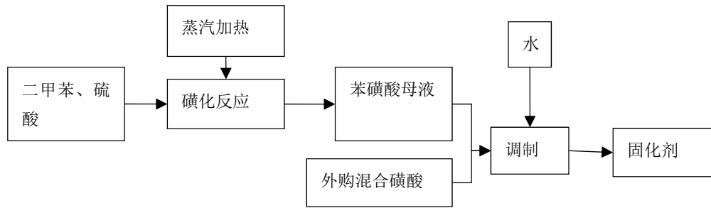
图 4.1-4 固化剂工艺流程工艺流程框图
