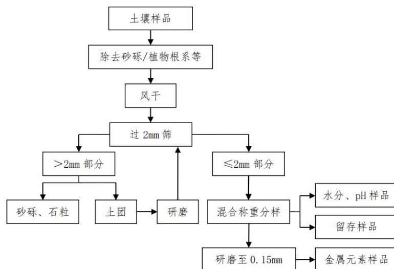
图 7.3-1 样品制备流程图
